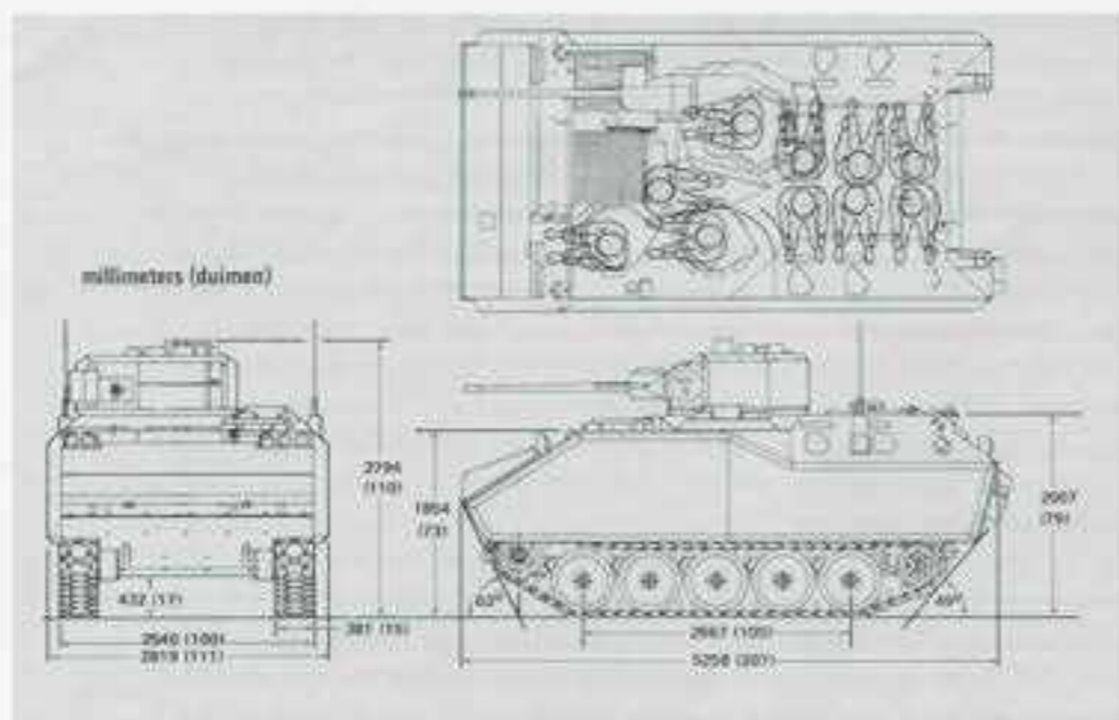
Afb. 5. Indeling YPR met maten. De plaats van de bestuurder is linksvoor. Daarachter zit de voertuigcommandant met naast hem in omgekeerde positie de plaatsvervangend voertuigcommandant en daarnaast de schutter. Commandant, chauffeur en schutter communiceren via de intercom. (Legerkoerier oktober 1977)
