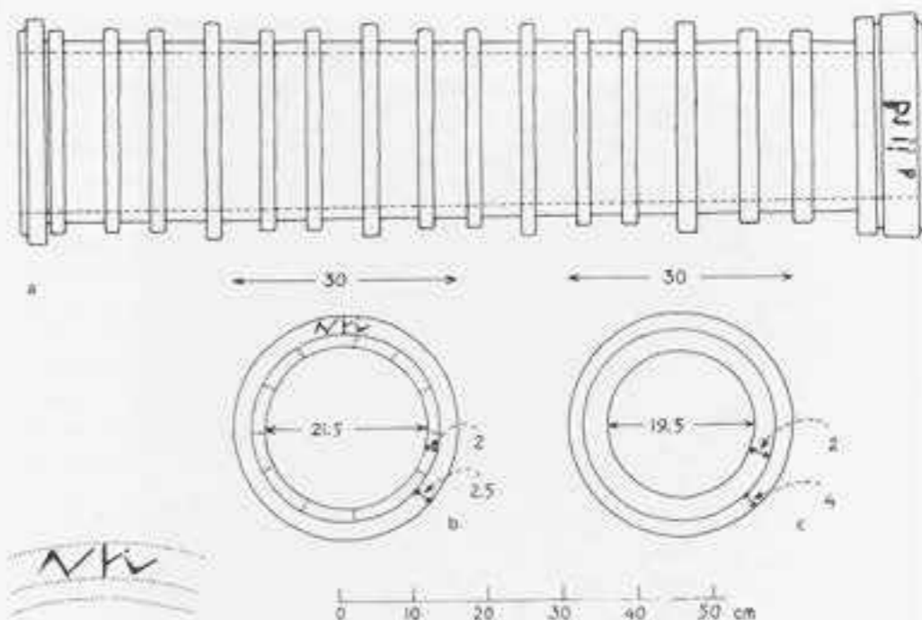
Afb. 7 Reconstructietekening van de Leuvense bombarde (Tekening J.P. Puype)
